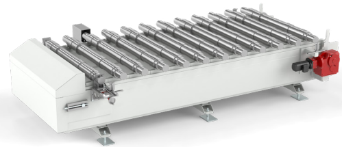
KETTENFÖRDERER FÜR ACHSEN
